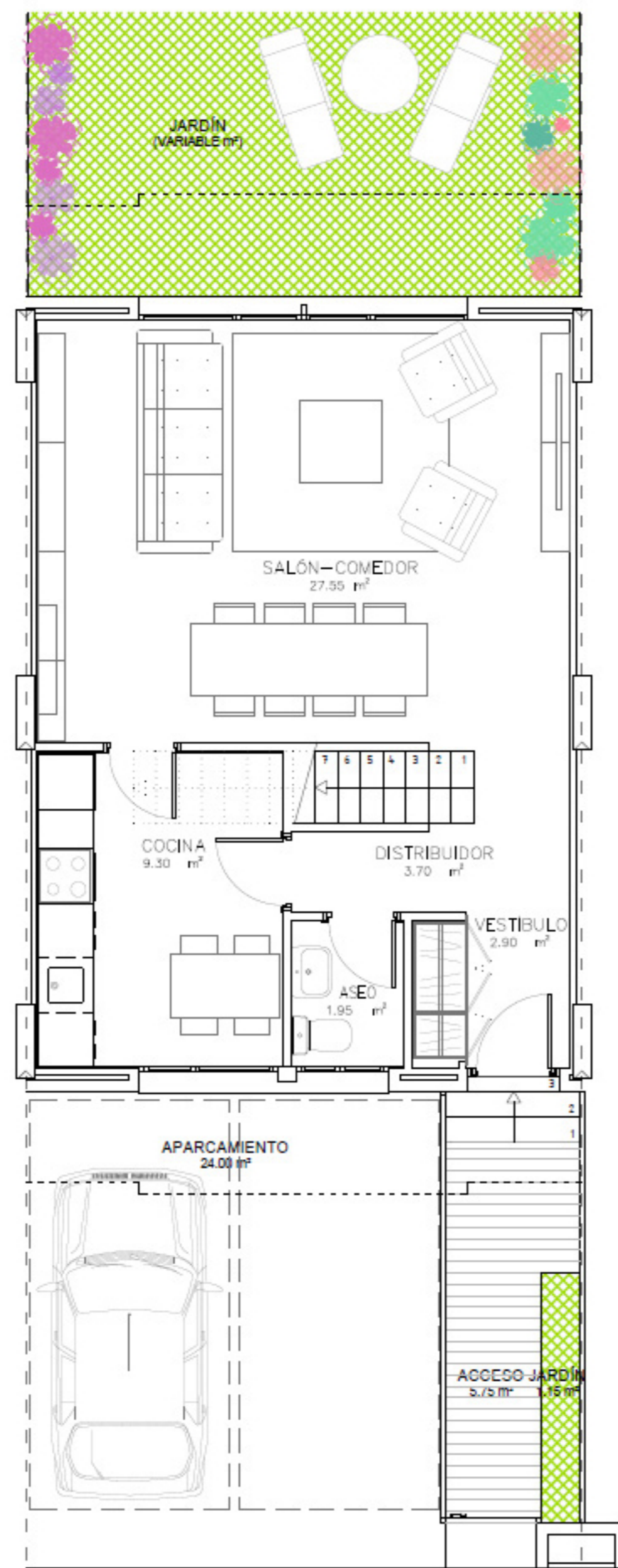
PLANTA BAJA
