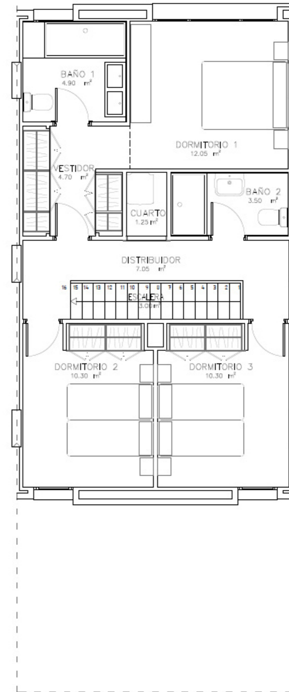
PLANTA PRIMERA
