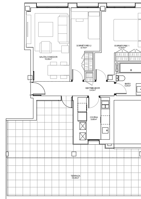
VIVIENDA TIPO 17 E=1/100
