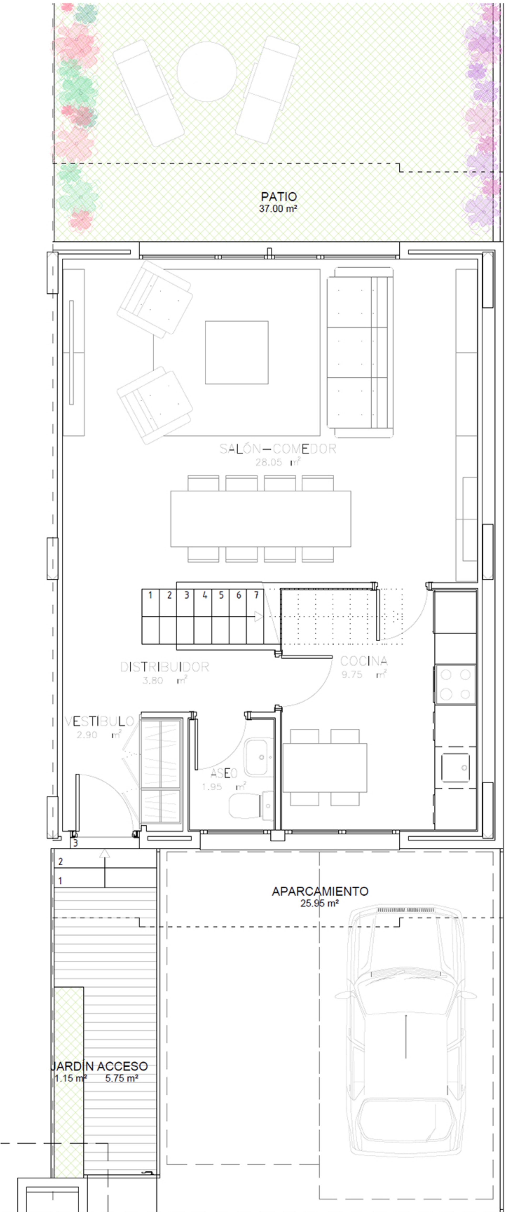
PLANTA BAJA
