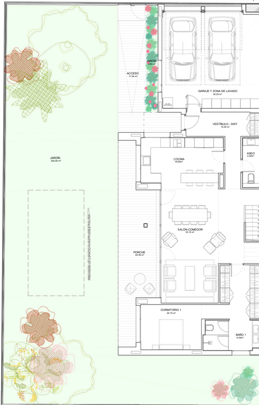
PLANTA BAJA
