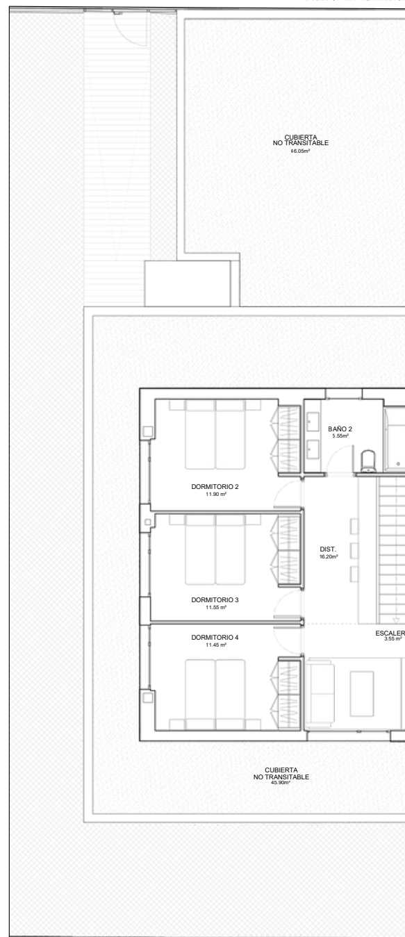
PLANTA PRIMERA
