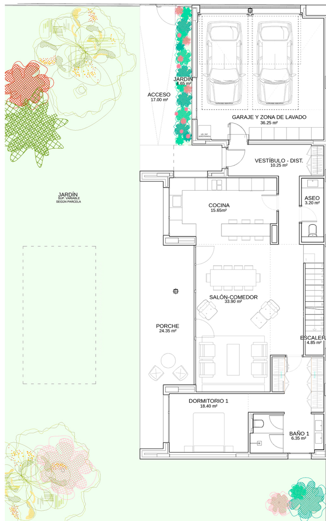
PLANTA BAJA [IZQUIERDA]
